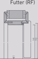
Vertikalschnitt Futter (RF)
