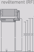
Coupe verticale du revêtement (RF)
